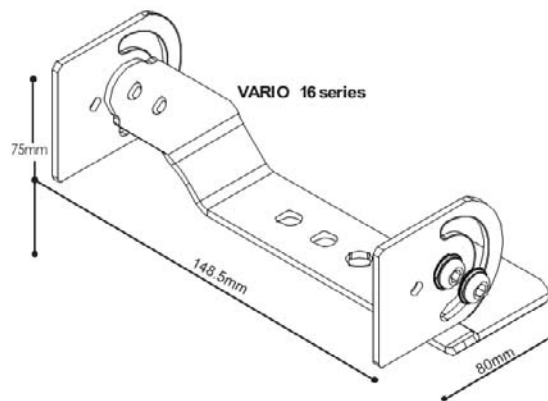
VUB-Plate
